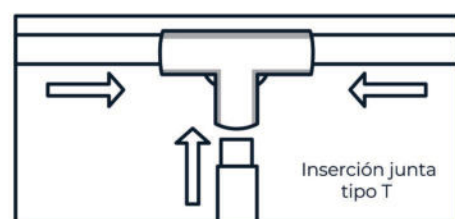
Método de instalación (Medio)
